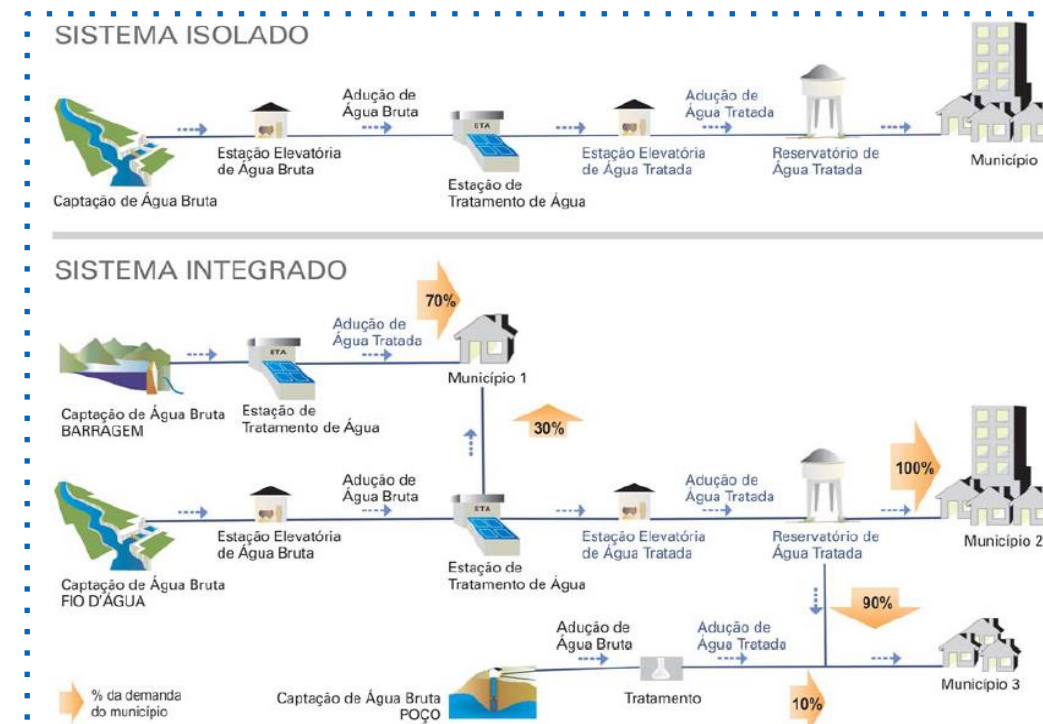
Ilustração simplificada do de sistemas de abastecimento
