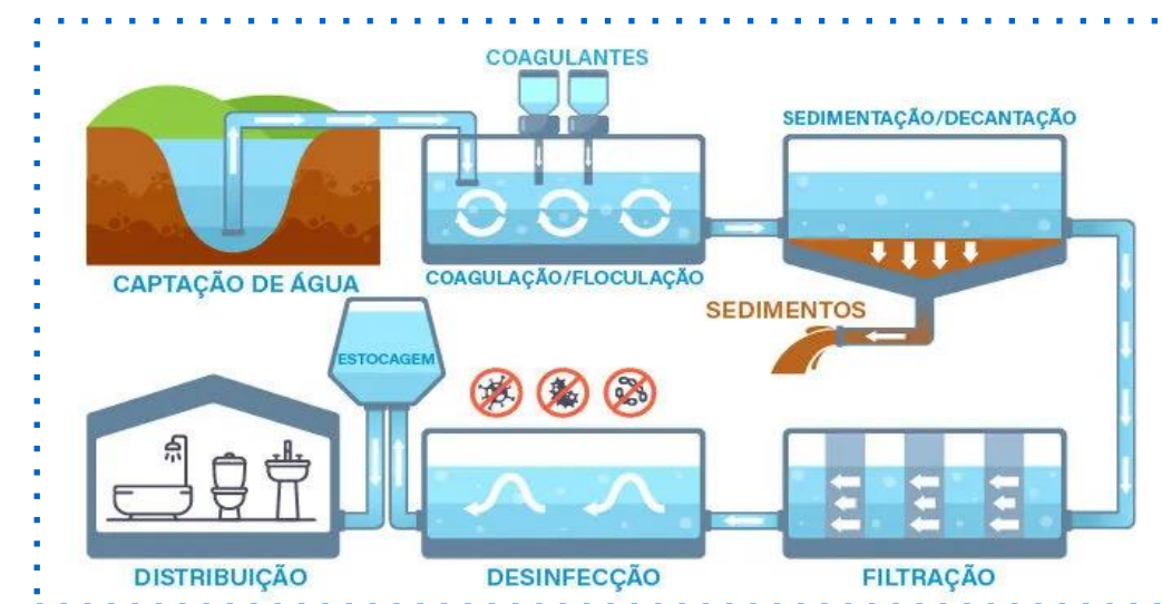
Ilustração simplificada do de sistemas de abastecimento
